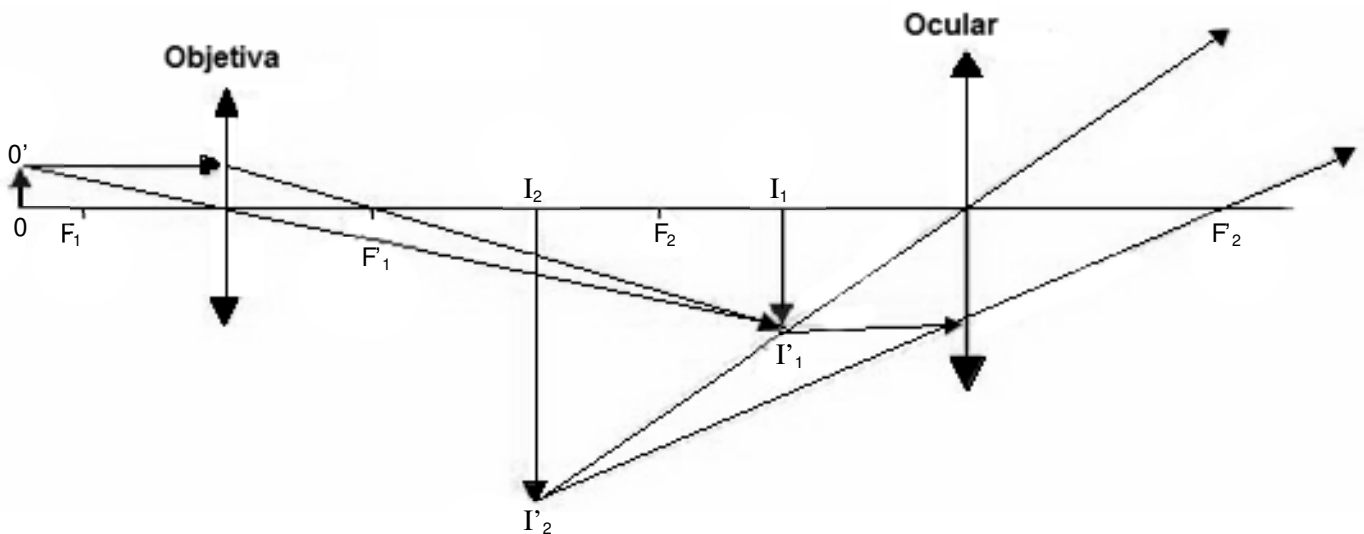
Figura: Diagrama esquemático da formação da imagem em um microscópio óptico.
